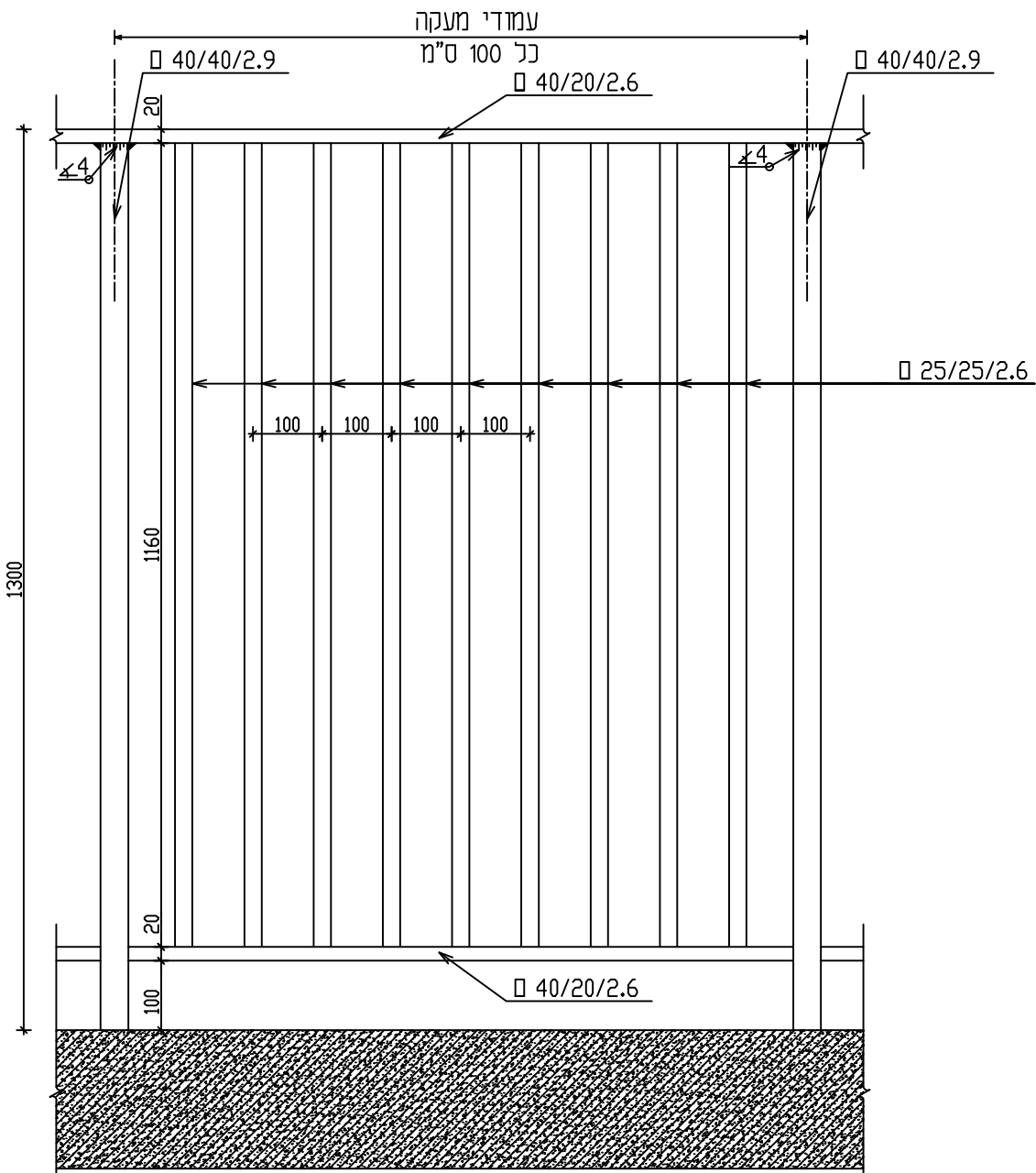
פרט מעקה טיפוסי 1:10
